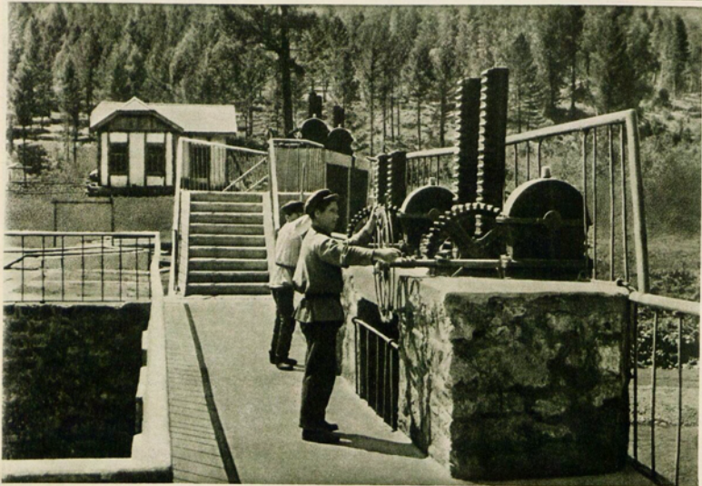
Убятская оросительная система.
