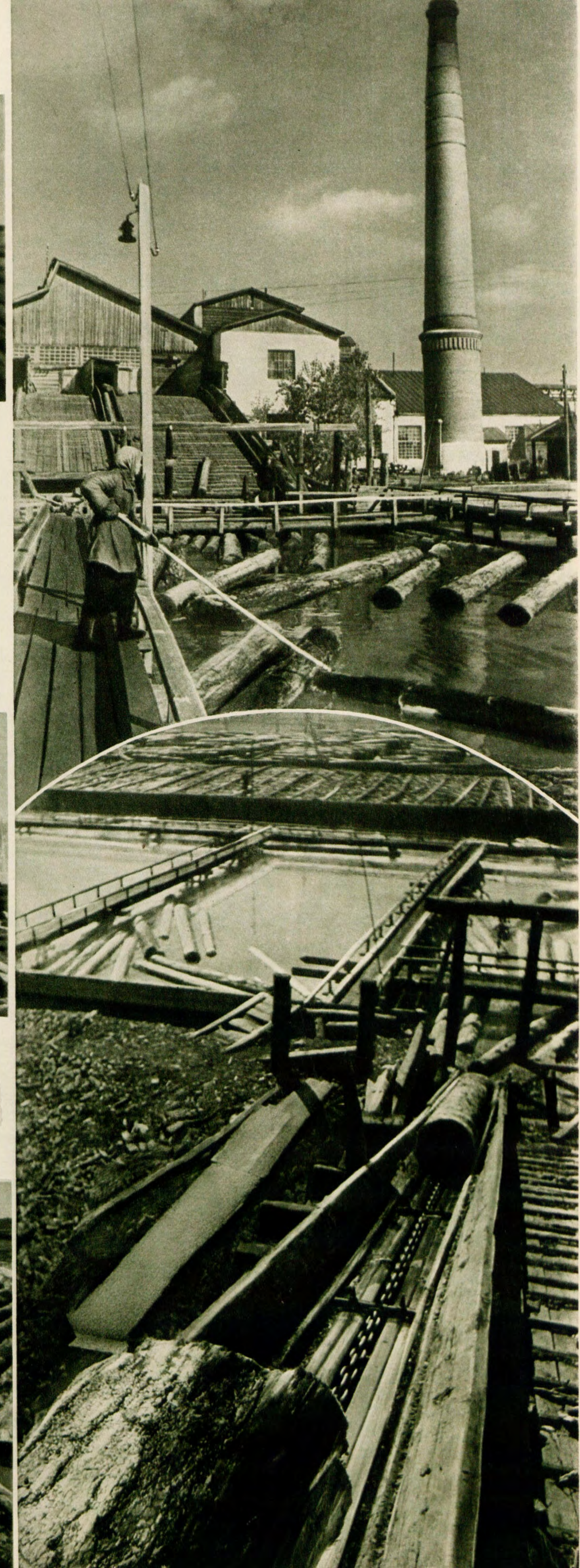
Абаканский деревообделочный комбинат. Подача конвейером бревен из бассейна к лесопильным рамам.
