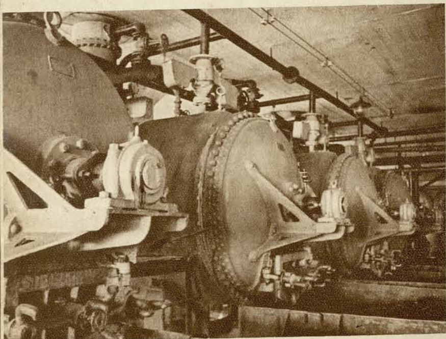
Котлы Лаабса.
