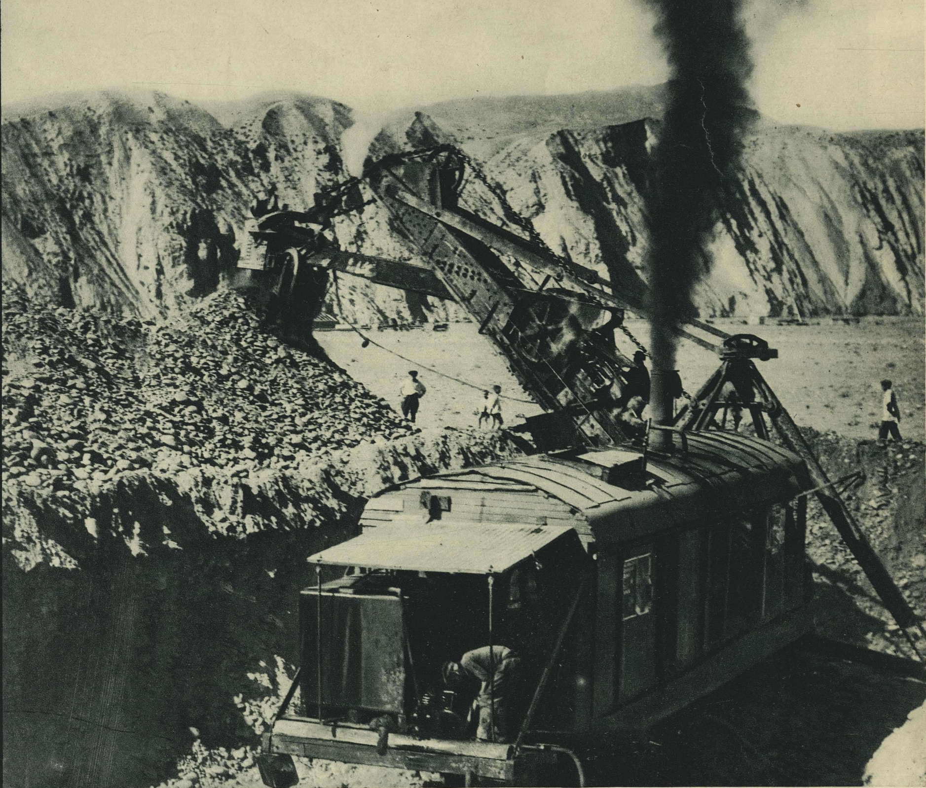
Подвозка камня для укрепления берега реки Вахш
