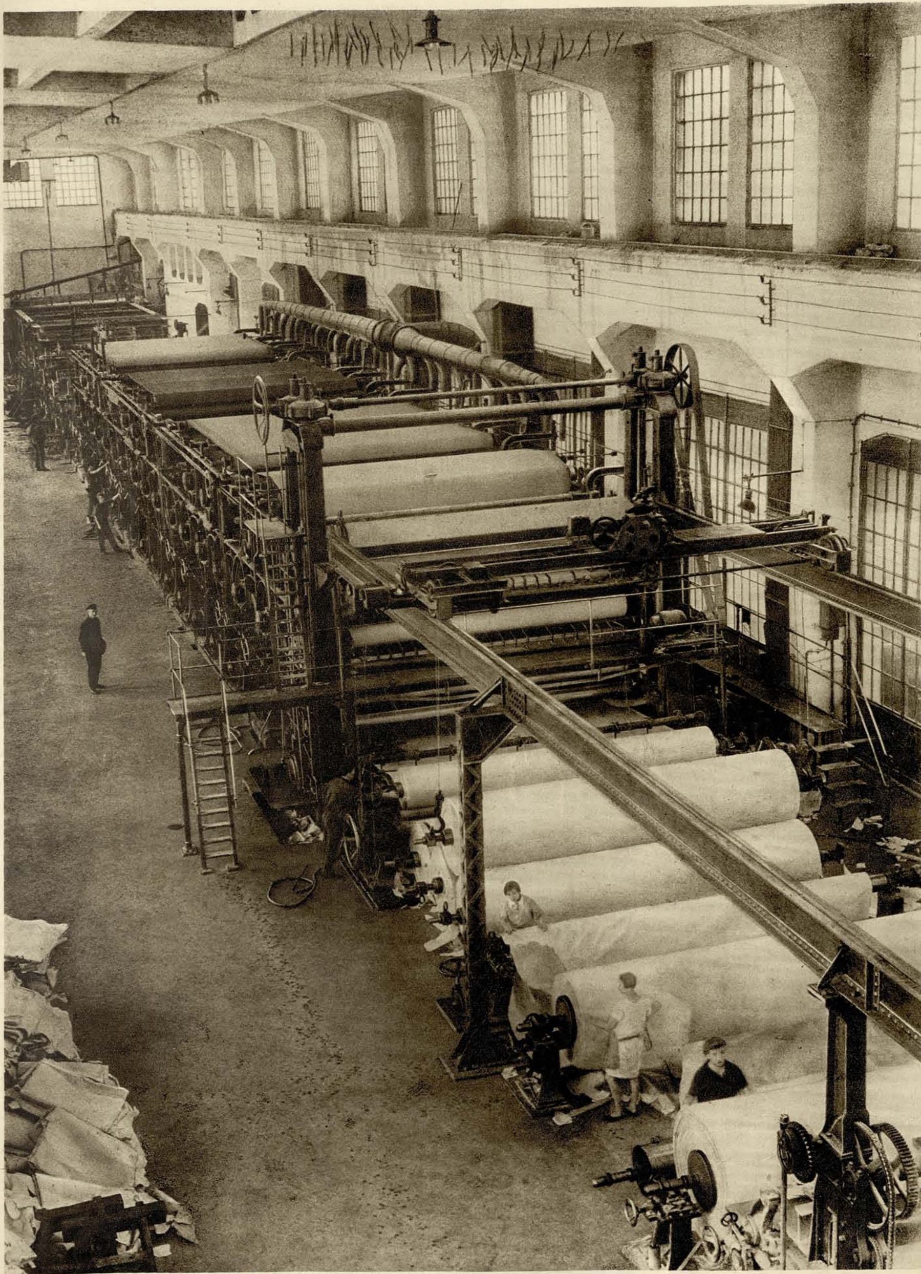
БУМАГОДЕЛАТЕЛЬНАЯ МАШИНА. ВИД СО СТОРОНЫ ВЫХОДА С МАШИНЫ ГОТОВОЙ ПРОДУКЦИИ
