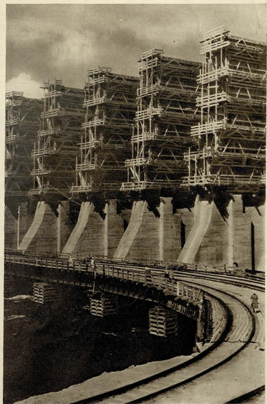
ЧАСТЬ ДНЕПРОВСКОЙ ПЛОТИНЫ
