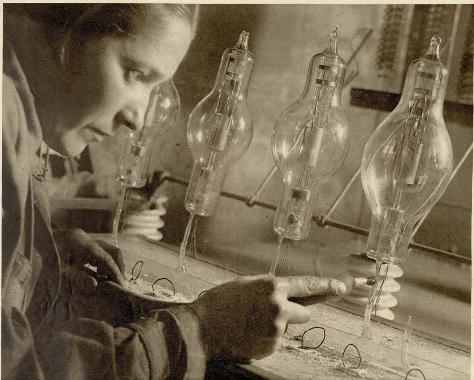
ЭЛЕКТРОЗАВОД В МОСКВЕ. ОТКАЧКА ГЕНЕРАТОРНЫХ ЛАМП В ЦЕХЕ ЭЛЕКТРОННЫХ ЛАМП
