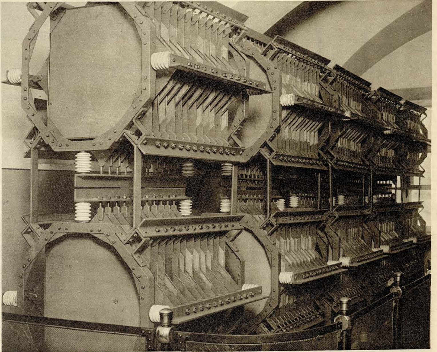
КОНДЕНСАТОРЫ ПОСТОЯННОЙ ЕМ- КОСТИ МОЩНОГО КАСКАДА НА РА- ДИОСТАНЦИИ ИМЕ- НИ КОМИНТЕРНА
