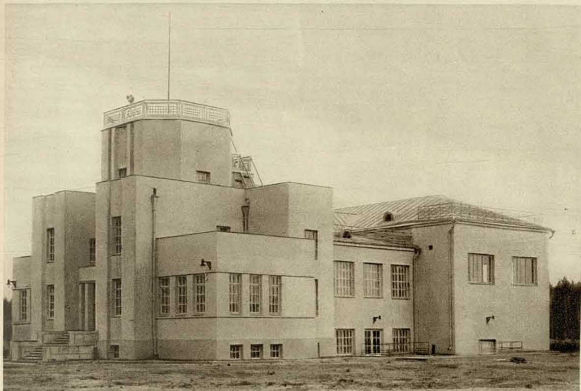
ЗДАНИЕ РАДИОСТАНЦИИ ВЦСПС В ЩЕЛКОВЕ ПОД МОСКВОЙ
