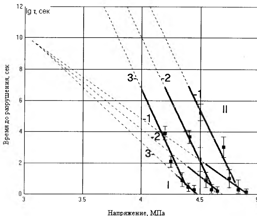
Зависимость долговечности мелкозернистого бетона от напряжения при водоцементном отношении 0.3 и цементнопесчаном отношении 1:1,2
