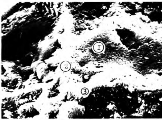
Рис. 1. Структура цементного камня –микробетона (3500х)
