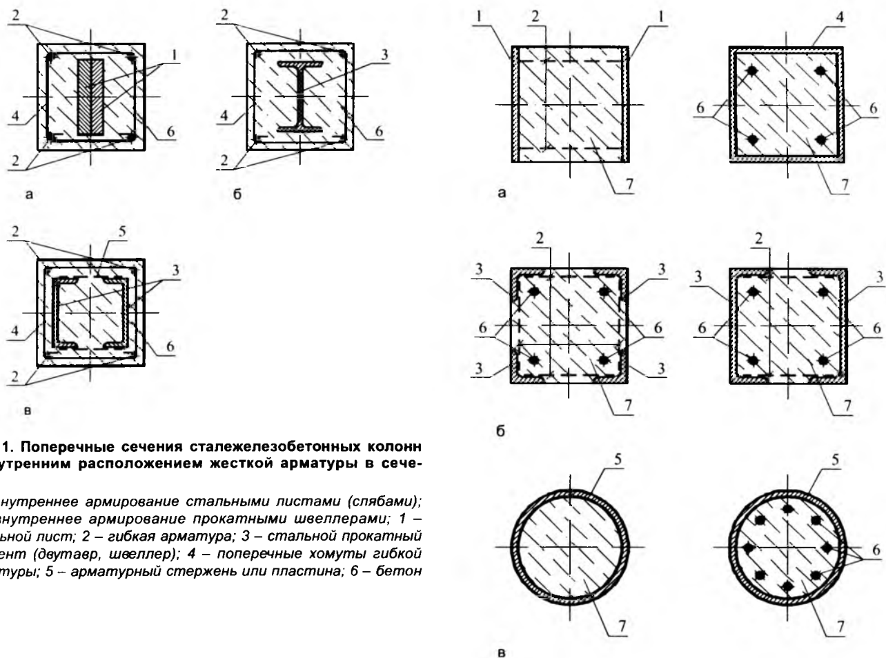
Рис. 2. Поперечные сечения сталежелезобетонных колонн с внешним расположением жесткой арматуры в сечении
