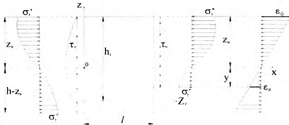
Рис. 1. Блок железобетонной балки
