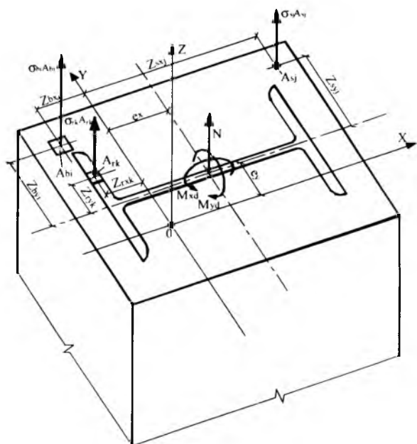
Рис. 3. Расчетная схема нормального сечения сталежелезобетонного элемента
