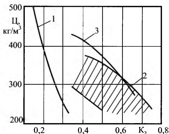
Рис. 3. Влияние расхода цемента на K_z по литературным данным:
