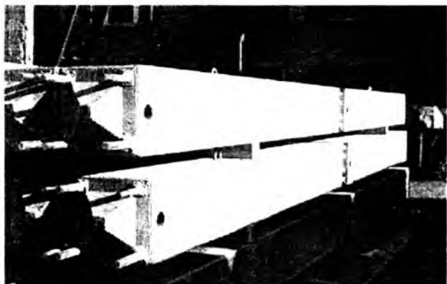
Рис. 3. Колонны сборно-монолитного безригельного каркаса системы КУБ-2,5
