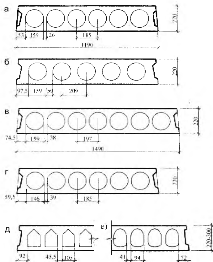
Рис. 1. Поперечные сечения многопустотных плит
