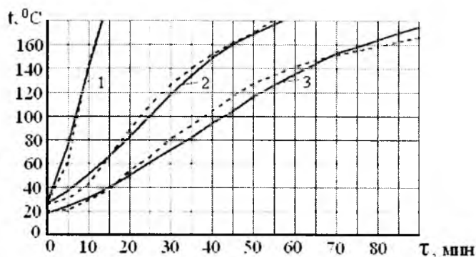
Экспериментальные (сплошные линии) и расчетные (пунктирные линии) кривые изменения температуры на необогреваемой поверхности плит
