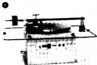
Круг истирания Беме, размеры 890x760x890 мм, масса 500 кг, 3/380 В
