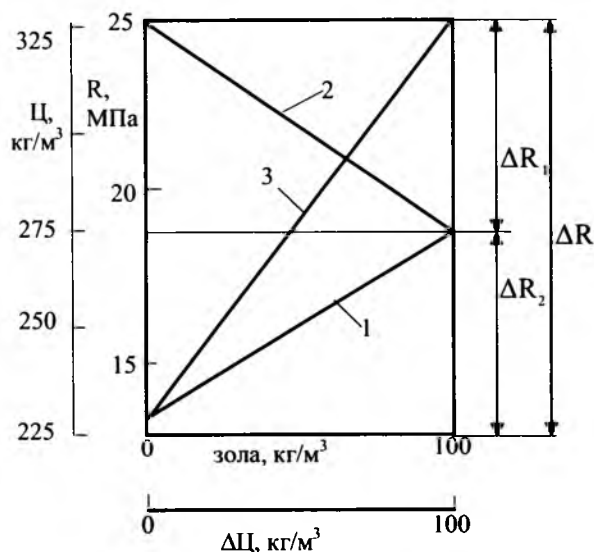
Рис. 1 Прочностные эффекты введения золы различными способами
