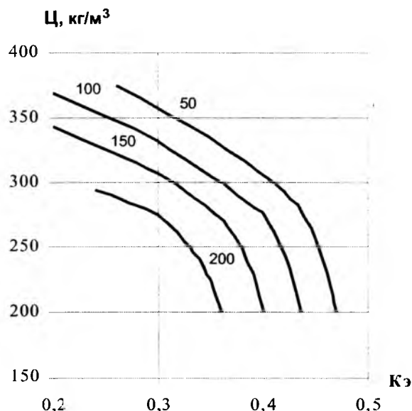
Рис. 2. Влияние расходов цемента и золы в бетоне на K_3
