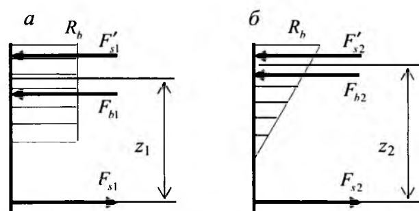
Схема усилий в сечении примера 4 [6] при расчете: а – по [2, 6], б – по [3, 4]
