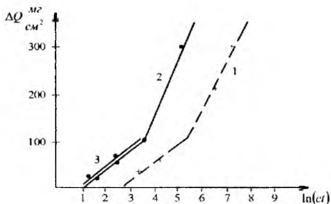
Рис. 7. Зависимость количества связанных ионов кальция (CaO) от количества раствора серной кислоты
