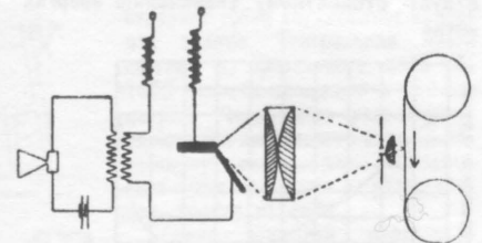
Схема установки Э. Румера
