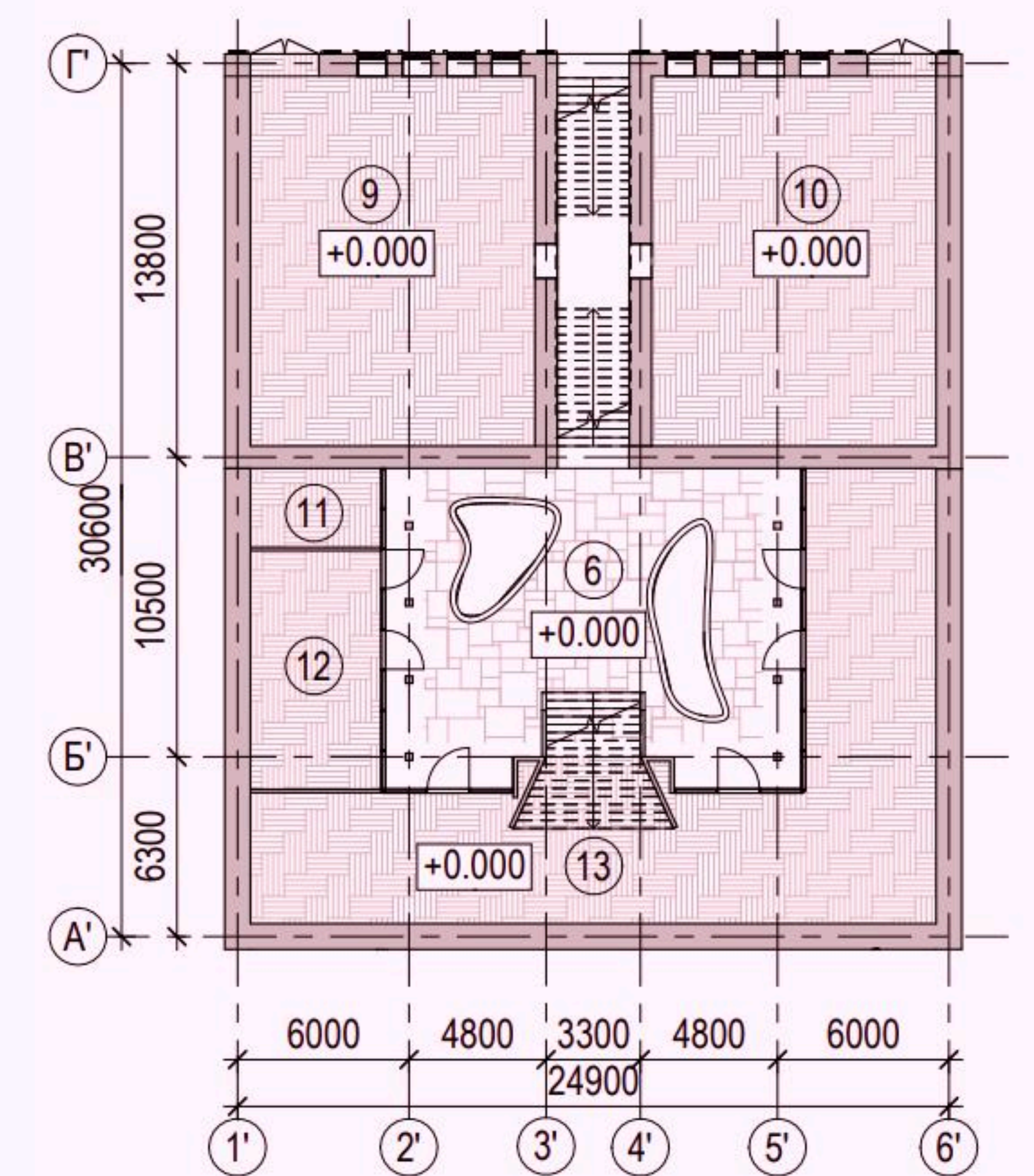
Планы первого и второго этажей дома на Киселёва 62
