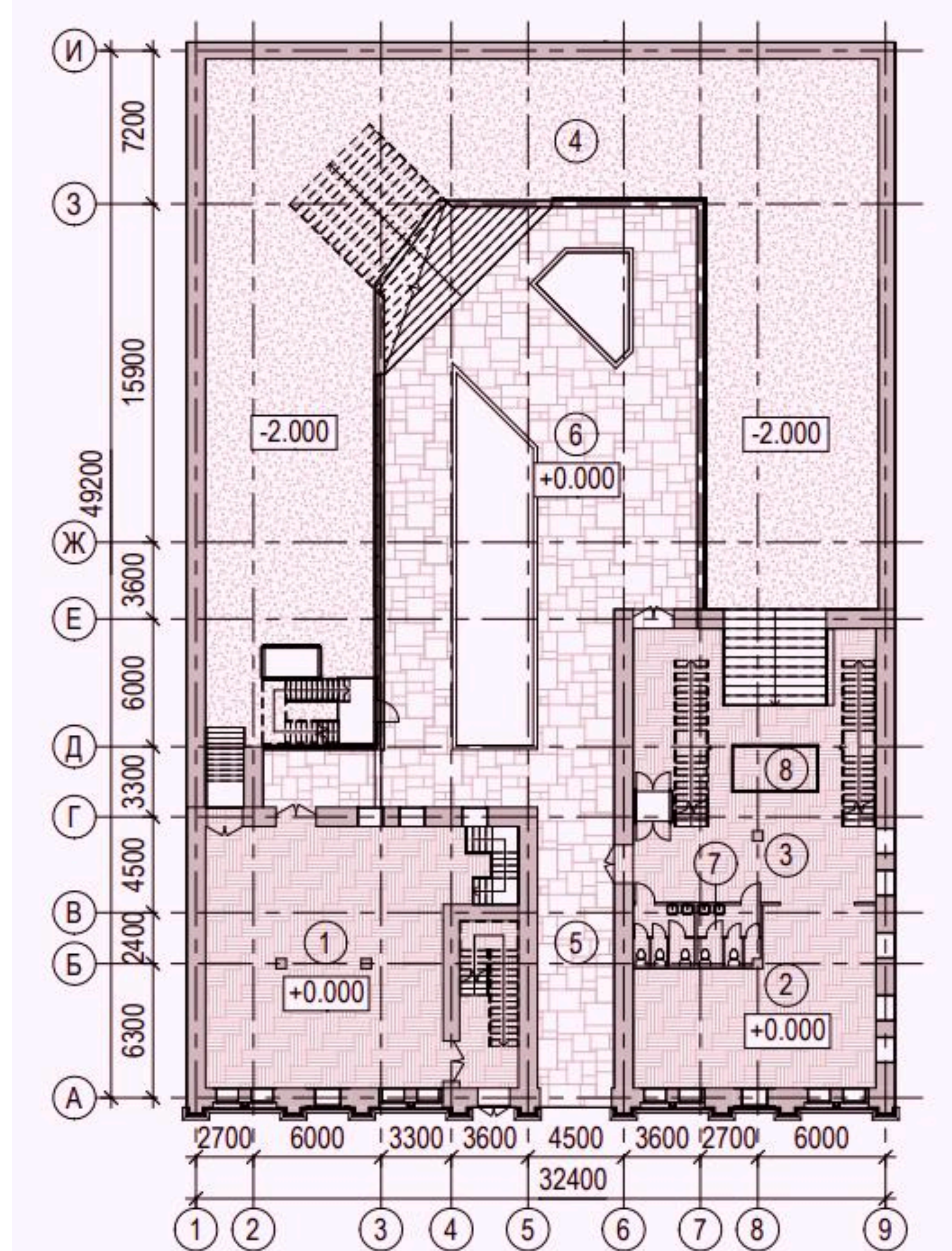
Планы первого и второго этажей "Дома художника"
