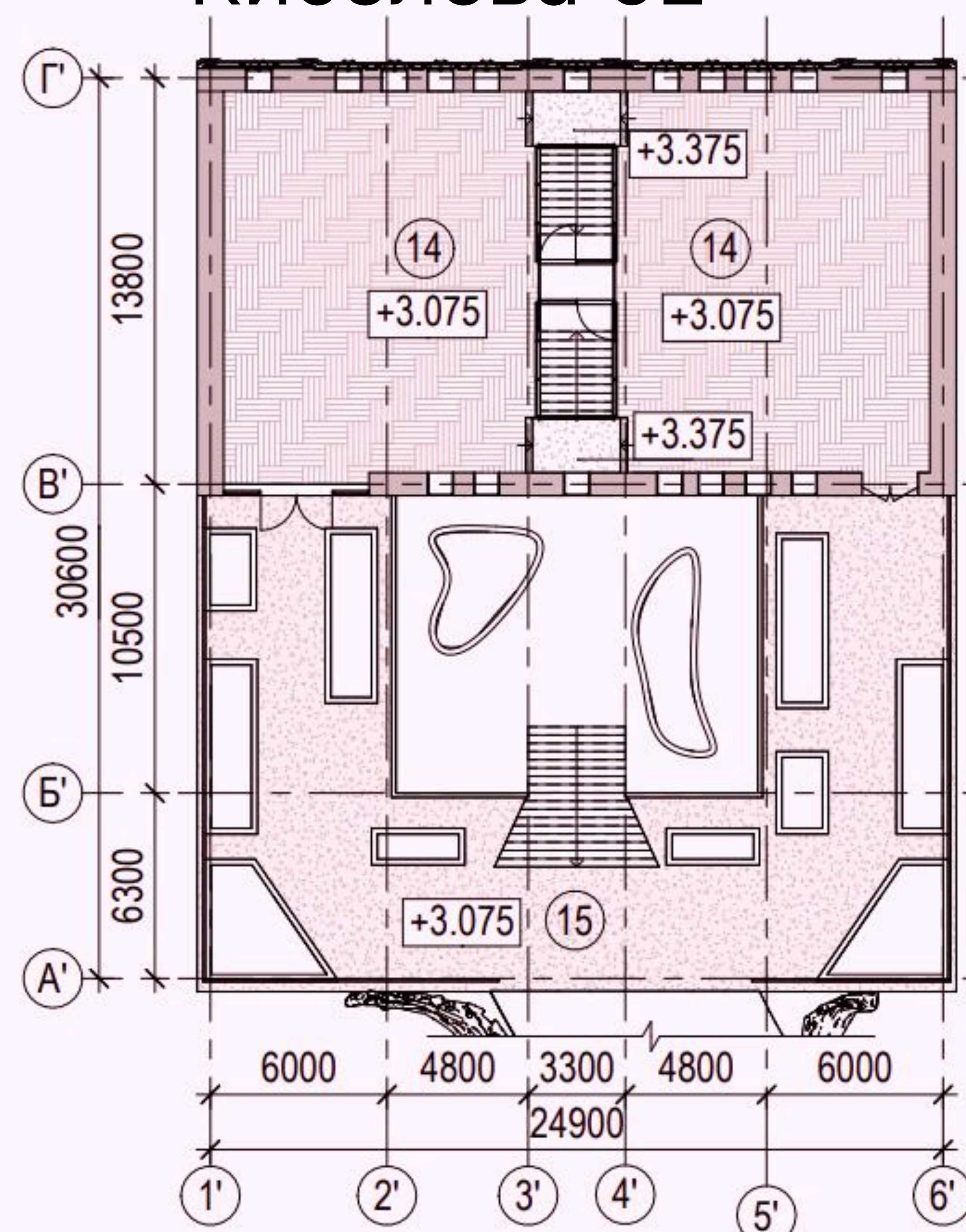
Планы первого и второго этажей дома на Киселёва 62
