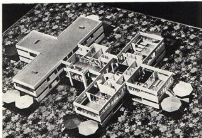
Типовой проект 212-2-65 яслей-сада на 280 мест. Макет и план первого этажа. Архитекторы Ф. Бабушкина, А. Михе, Ю. Шаронов
