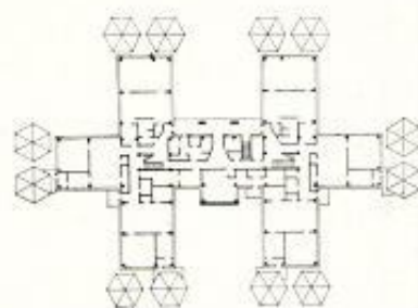
Типовой проект 212-2-65 яслей-сада на 280 мест. Макет и план первого этажа. Архитекторы Ф. Бабушкина, А. Михе, Ю. Шаронов
