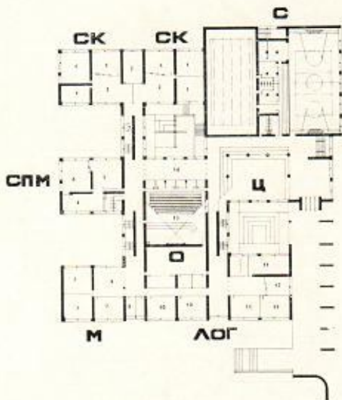
Проект школы на 30 классов для г. Кирова. Макет и план второго этажа. ЦНИИЭП учебных зданий. Архитекторы: В. Степанов, А. Степанов, К. Френкель
