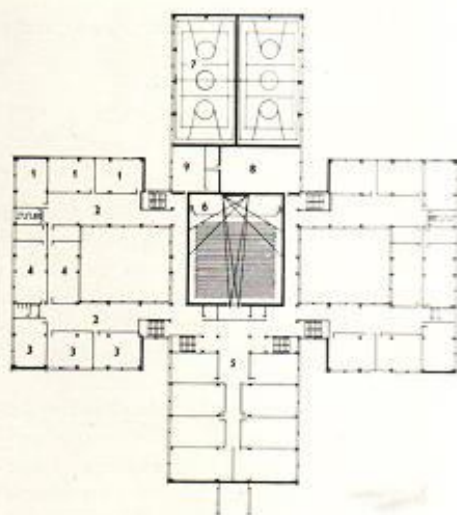
Школьный комплекс на 30+30 классов. ЦНИИЭП учебных зданий. Архитектор А. Степанов. Фасад, план третьего этажа
