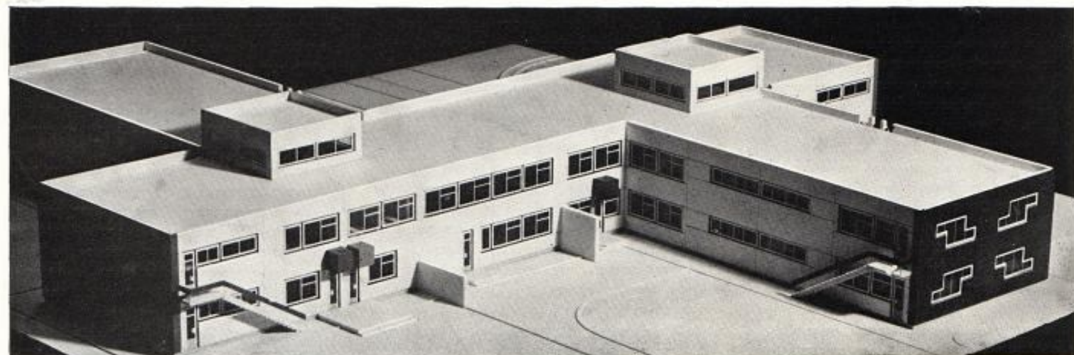
Типовой проект 211-2-108 яслей-сада на 320 мест в каркасно-панельных конструкциях серии ИИ-04. Архитекторы: Ю. Иванов, Р. Голышко, инженеры: Г. Гофман, Н. Быков
