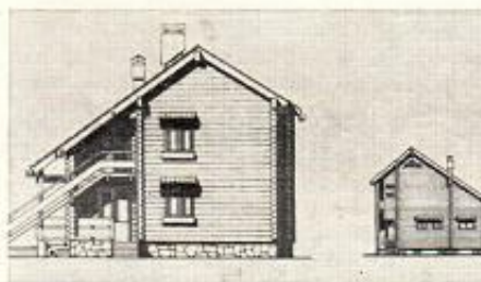
Р. Валиахметов, Д. Сафин. Конкурсный проект одноквартирного дома с рублеными стенами
