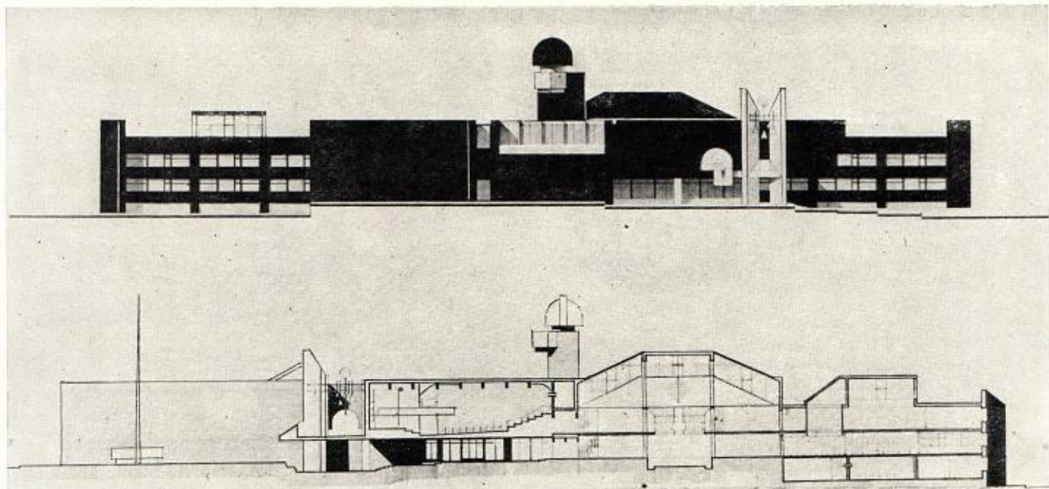
Проект школы на 33 класса для села Шали Татарской АССР. ЦНИИЭП учебных зданий. Архитекторы: А. Степанов, В. Степанов, К. Френкель Фасад и разрез
