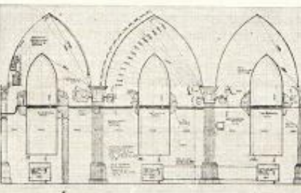
Г. Вязунова. Реконструкция и приспособление под зал органной музыки польского костела в Иркутске
