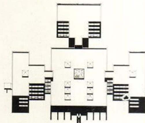
Школьные комплексы из функциональных блоков. Всесоюзный конкурс 1978 г. Премия. Архитектор А. Степанов. План этажа школьного комплекса на 30+30 классов.
