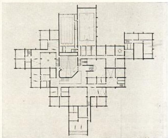
Проект школы на 31 класс в поселке Волосово Ленинградской области. Фасад и план второго этажа (варианты). ЦНИИЭП учебных зданий. Архитекторы: В. Степанов, В. Тирский, Л. Шалов
